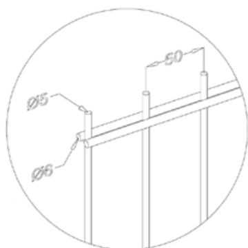
Dostępne wielkości paneli
