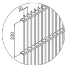
Rozstaw prętów
