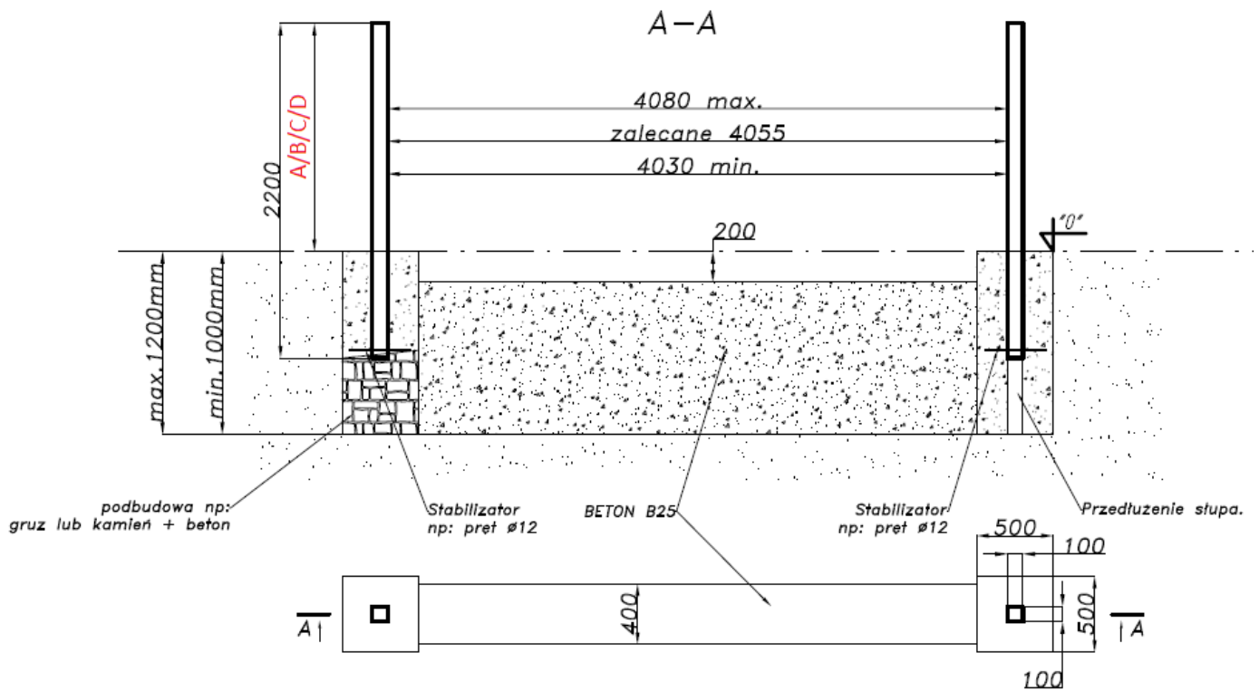
Rys. 2. Fundamenty bramy dwuskrzydłowej; wymiary: A- 1350 mm (Torino), B- 1400 mm (Bergamo), C- 1450 mm (Modena, Roma), D- 1500 mm (Ancona, Parma, Milano, Genua)
