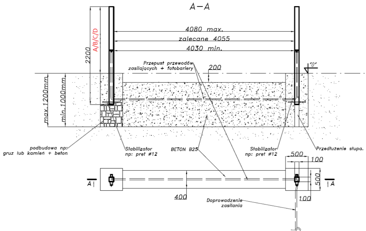
Rys. 6. Fundamenty bramy dwuskrzydłowej; wymiary: A- 1350 mm (Torino), B- 1400 mm (Bergamo), C- 1450 mm (Roma), D- 1500 mm (Ancona, Parma, Milano, Genua)
