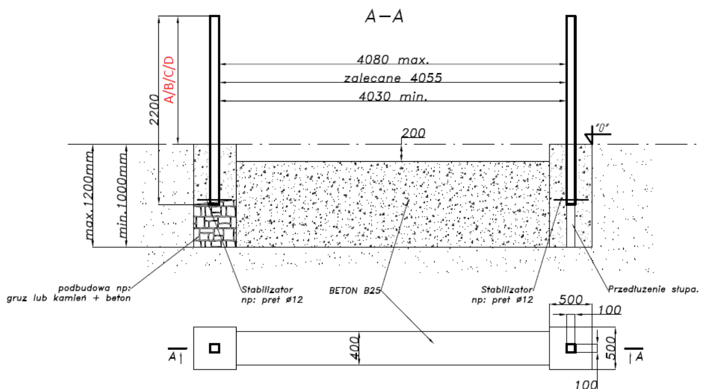
Rys. 2. Fundamenty bramy dwuskrzydłowej; wymiary: A- 1350 mm (Torino), B- 1400 mm (Bergamo), C- 1450 mm (Rimini, Roma), D- 1500 mm (Ancona, Parma, Milano, Genua, Treviso)
