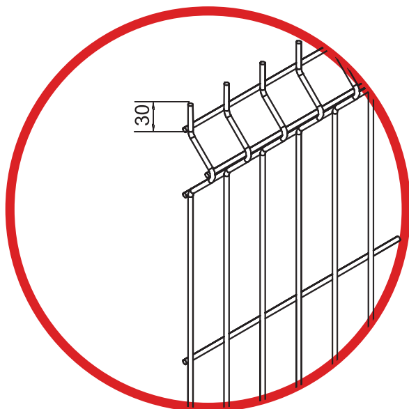
Górna krawędź standard wystający drut do 30 mm
